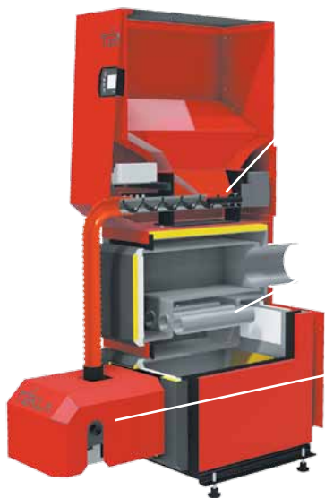
FIREBLAST automata pellet égőfej
